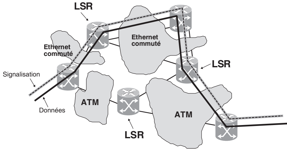
Figure R.5 Réseau MPLS de transition
