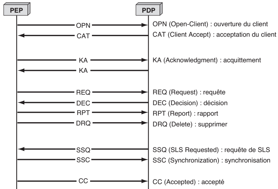
Figure S.20 Échange de messages dans une communication COPS
