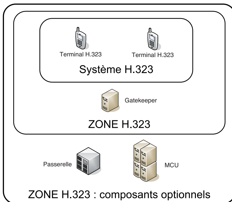
Figure T.6 Système et zones H.323
