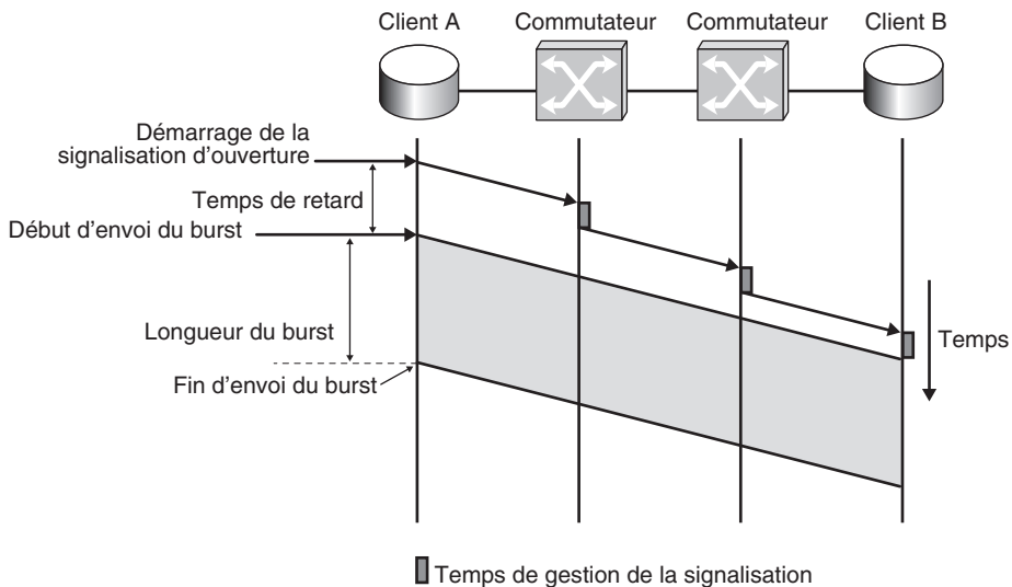
Figure J.7 Commutation par burst JIT et JEN
