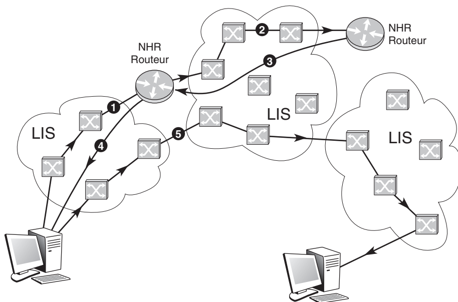
Figure L.8 Mise en place d'une route par NHRP
