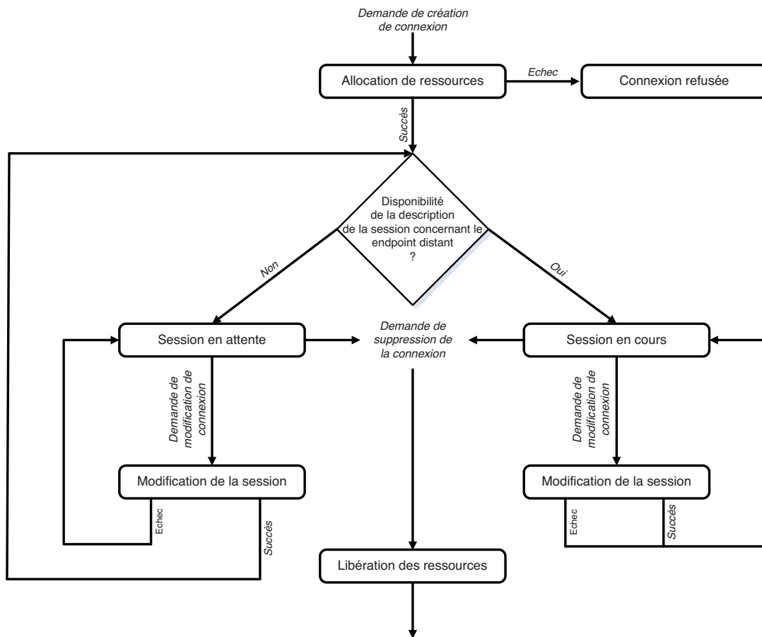
Figure T.18 Diagramme d'états d'une passerelle
