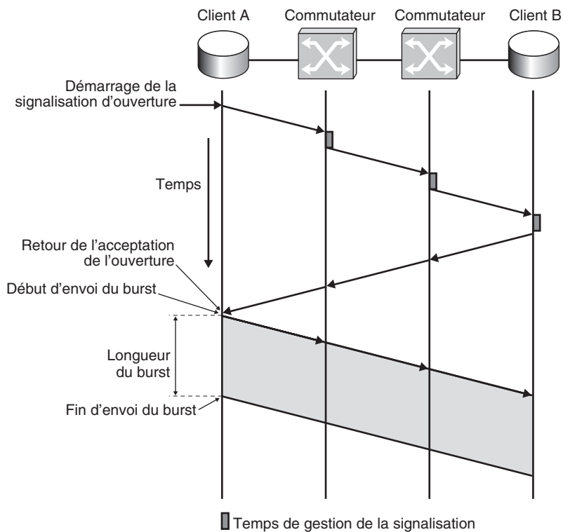
Figure J.6 Commutation par burst TAW
